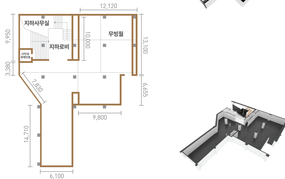
세종미술관 2관 도면 높이 2,850mm
